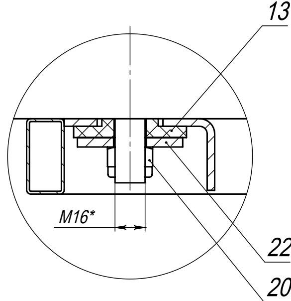
Д-Д (1 : 2)
