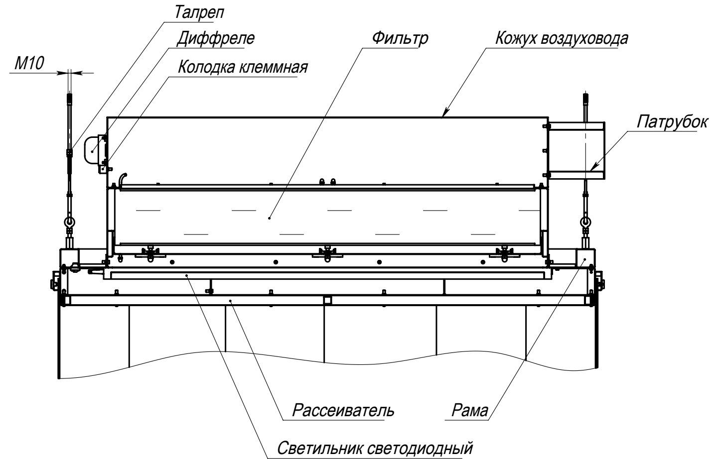
A-A (1 : 10)
