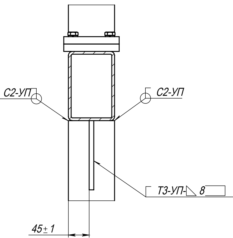
B-B (1 : 5) 2 места
