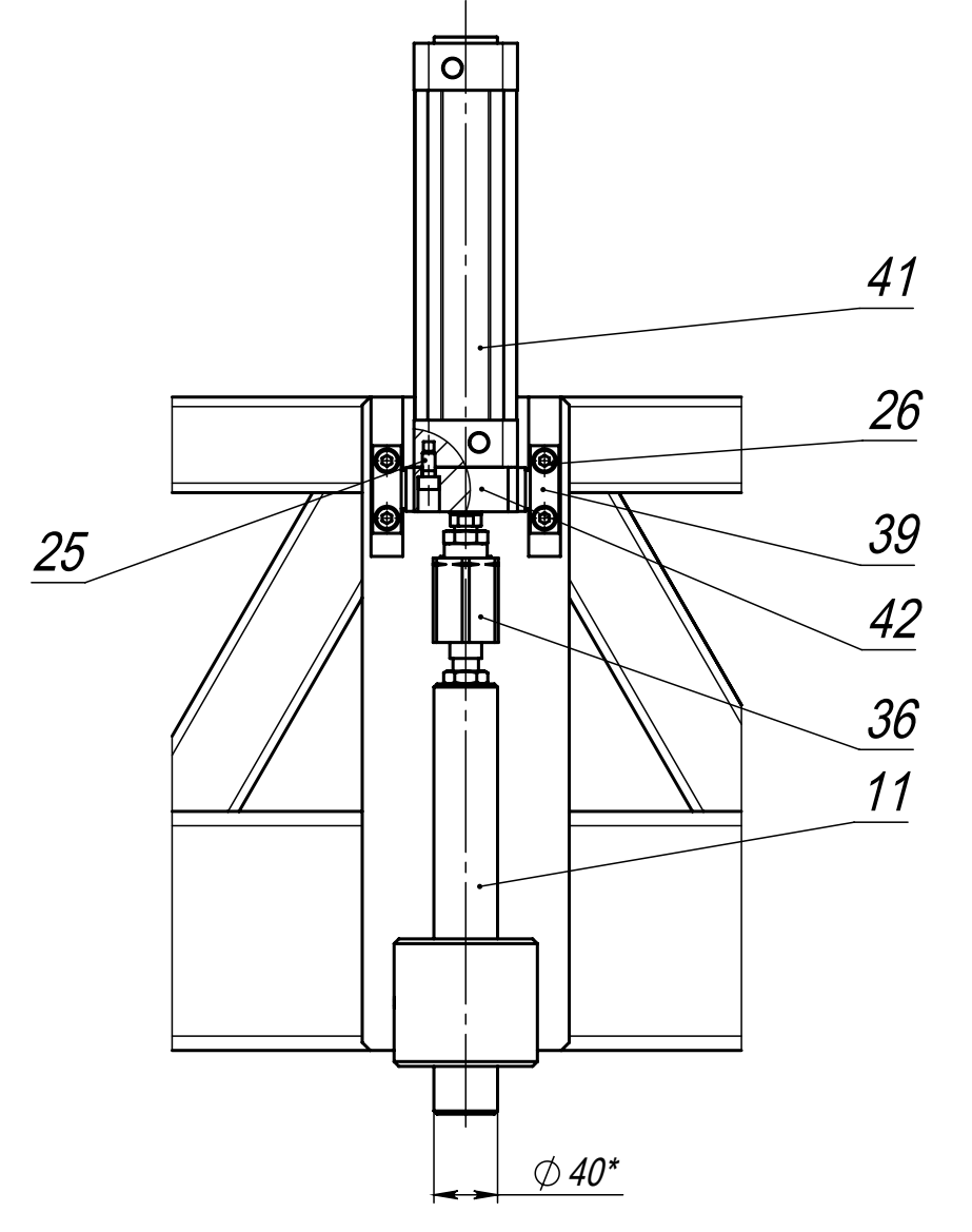
Д (1:5)
