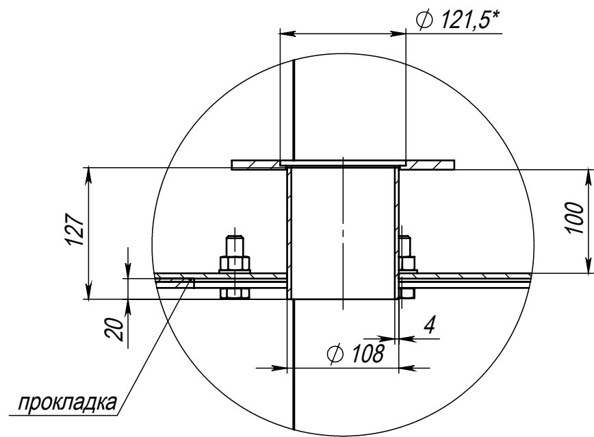
Б-Б (1 : 5)
