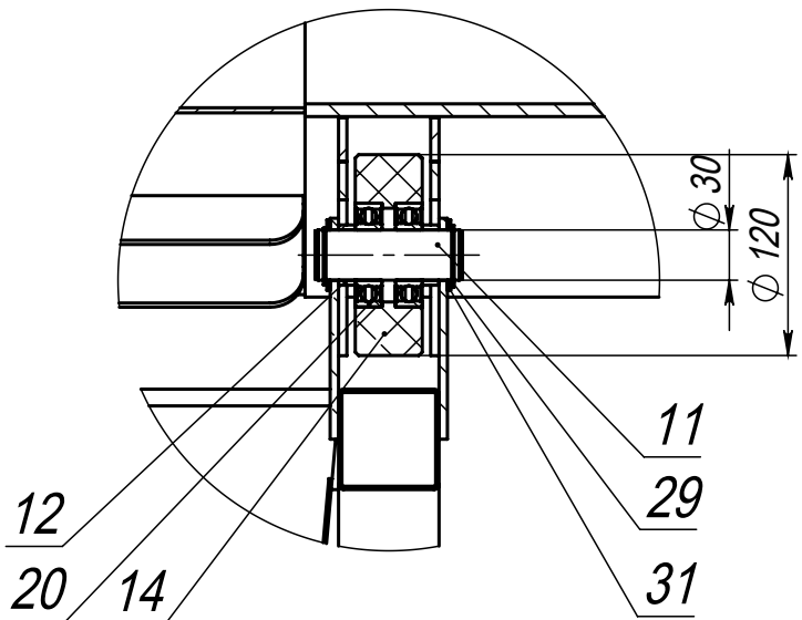
А-А (1 : 5)
